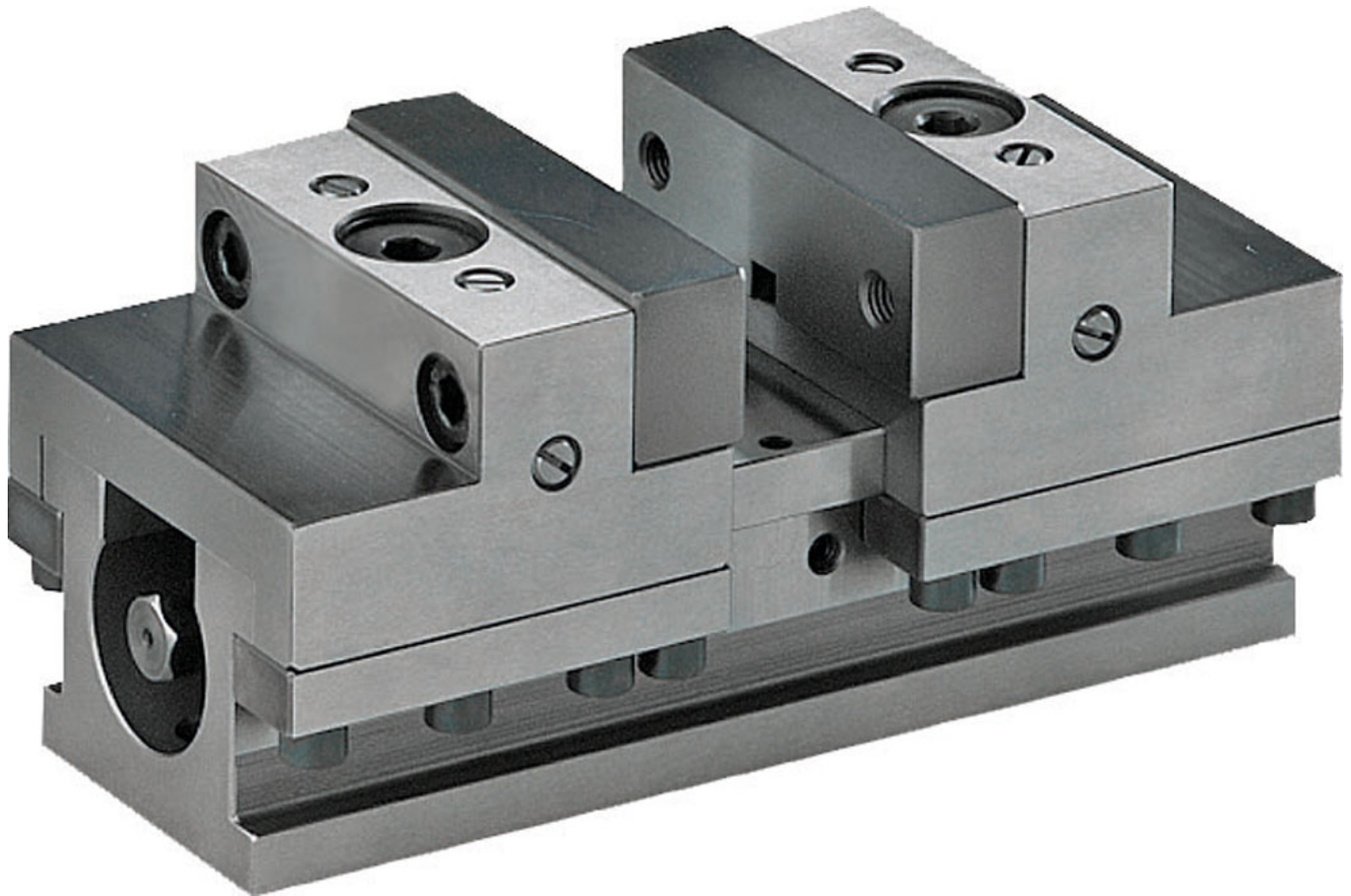
Mechanischer Zentrischspanner MZS Ausführung B mit weichen Spannbacken
