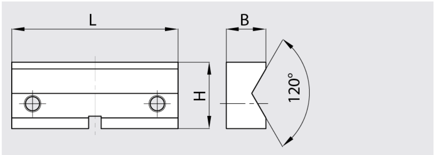
Planzeichnung Prismenbacken
