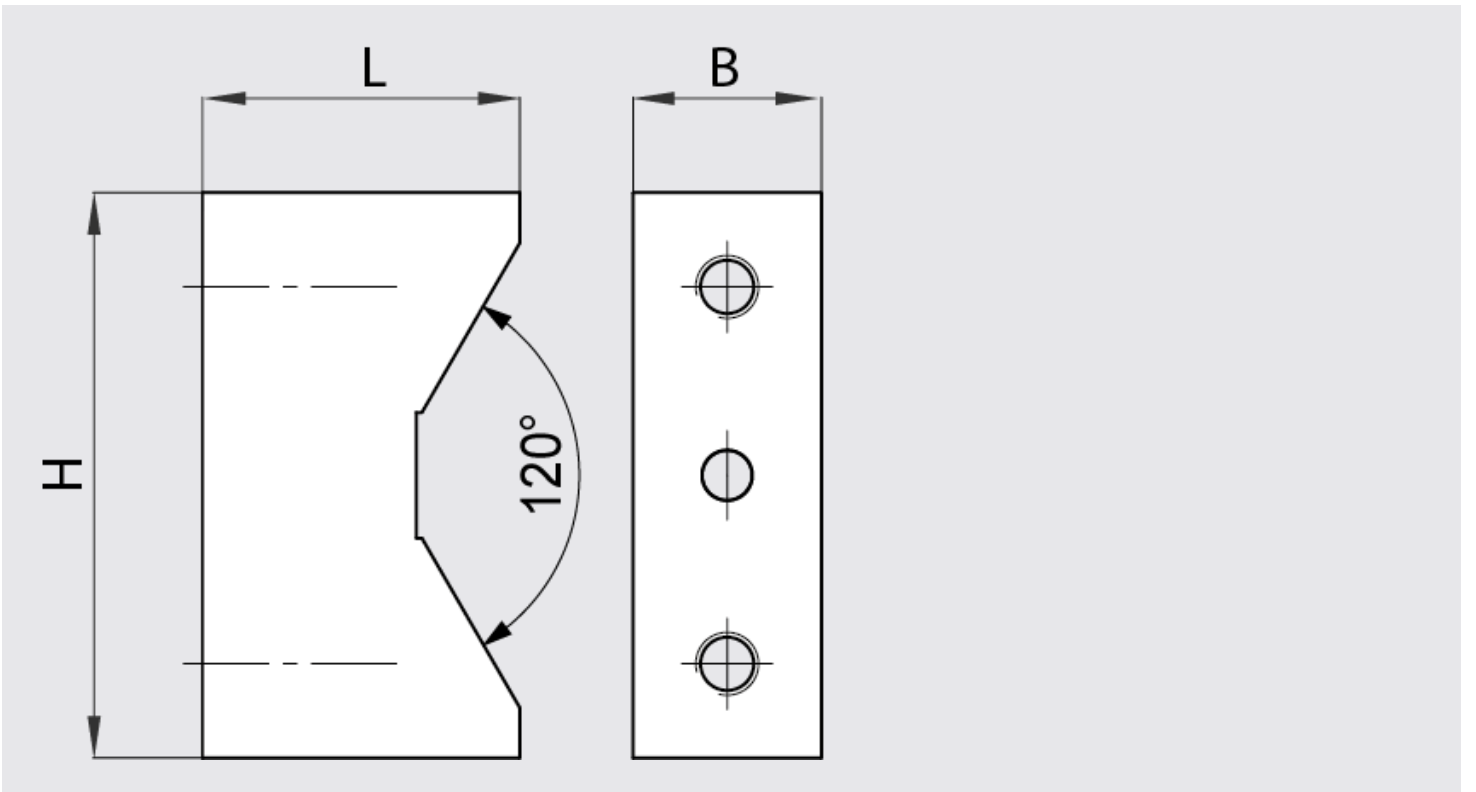
Planzeichnung Prismenbacken
