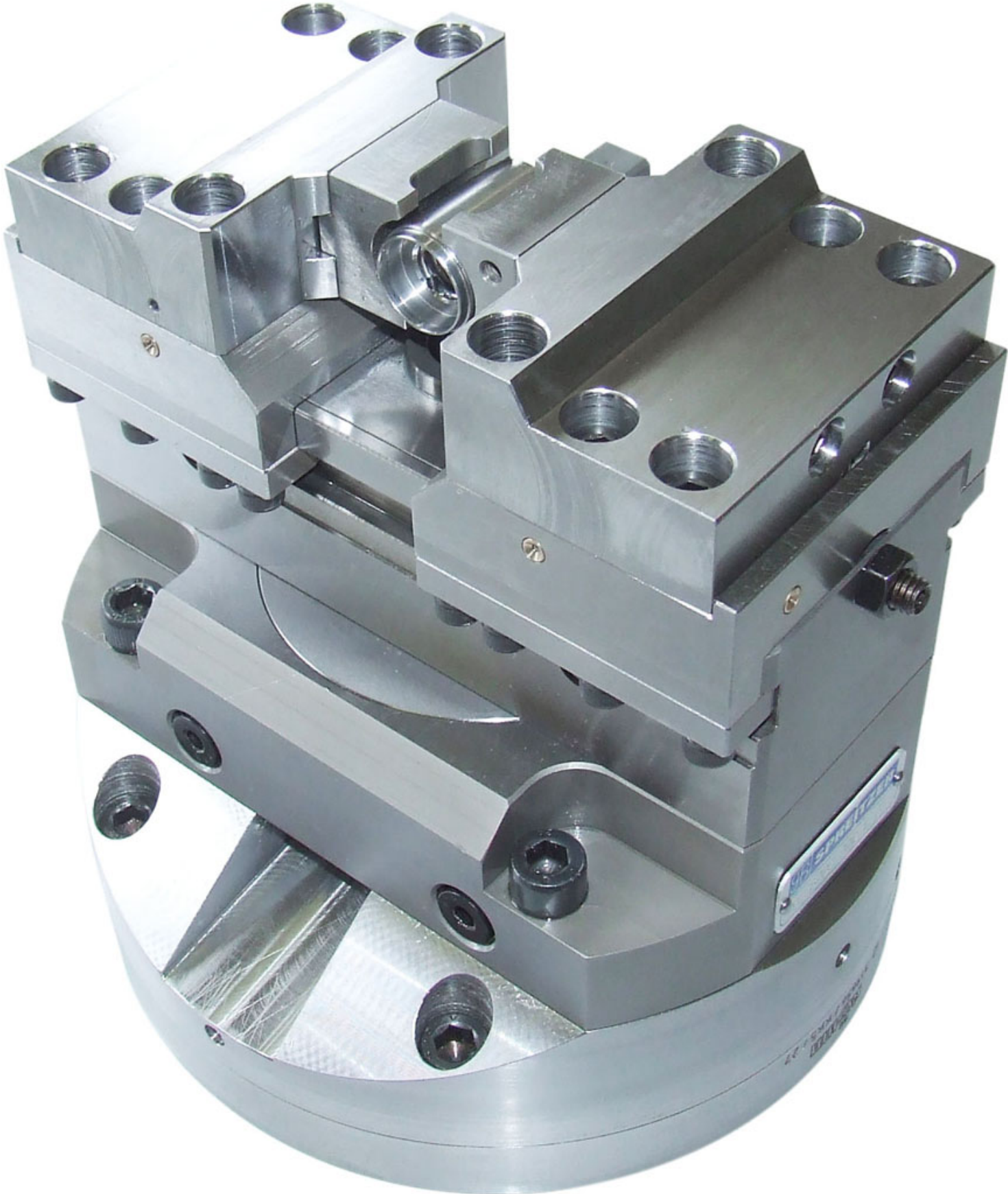
Kundenspezifische Prismenbacken
