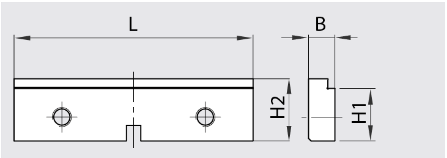
Maße Stufenbacken
